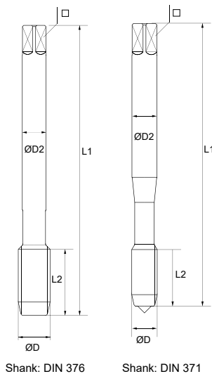
Shank: DIN 376
