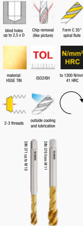
Shank: DIN 371
